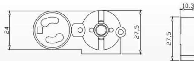
HC-19B(G13)
