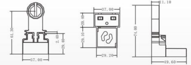
HB-39B(G13)
